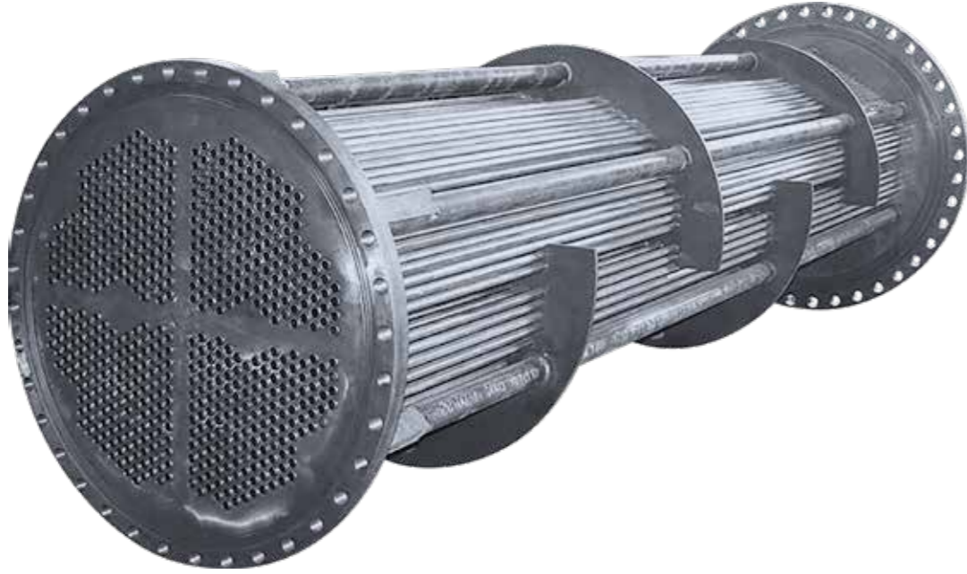
رادیاتور صنعتی | بندل آب گرم واحد نمکزدایی
