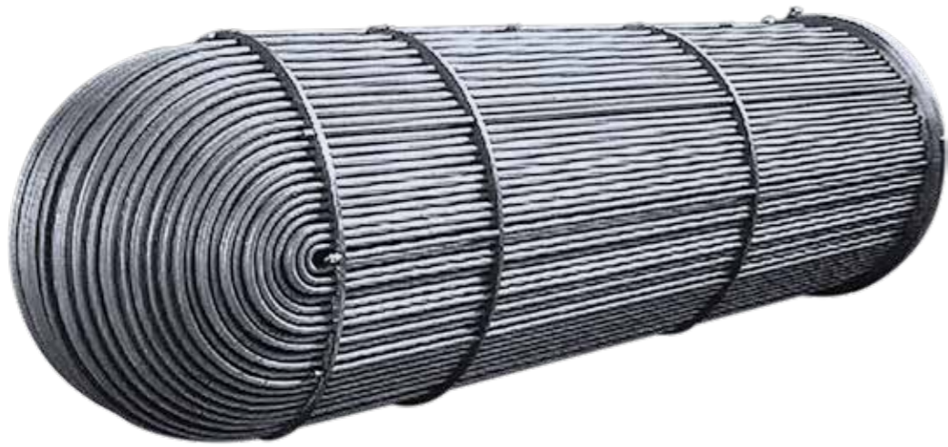
رادیاتور صنعتی | تیوب بندل
